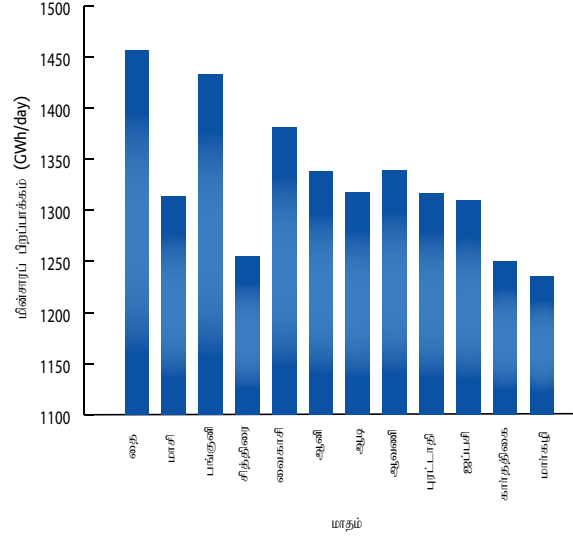
உரு T3: மாதாந்த மின்சாரப் பிறப்பாக்கம் (நிகர) - 2022
