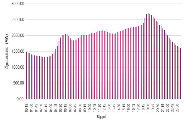
உரு T5: முறைமை மின் பிறப்பாக்க விபரம் - 2022-01-31 இல்
