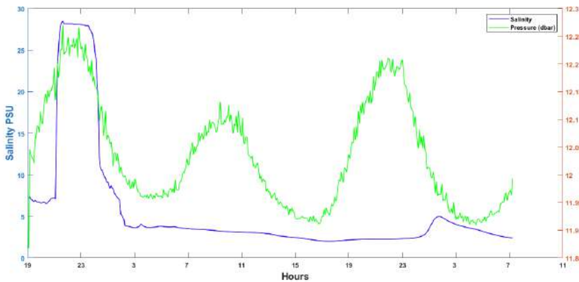
படம்23: மார்கழியில் கடல் மட்ட மாற்றங்களுடன் களப்பு வாய் உப்புத்தன்மை மாறுபாடு
