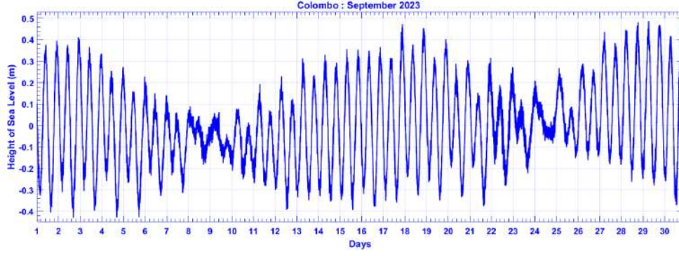
படம் 01: கொழும்பில் கடல் மட்ட மாறுபாடு
