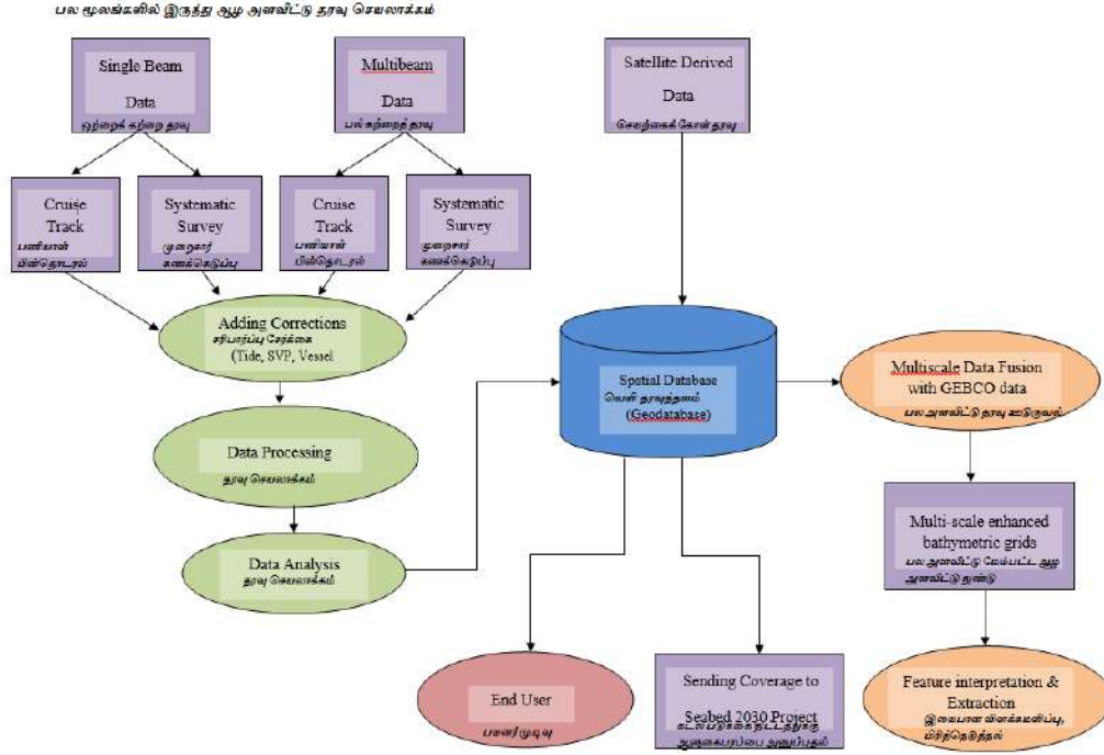
படம் 2.1: பல மூல தரவு செயலாக்கத்தின் செயல்பாட்டு செயல்முறை
