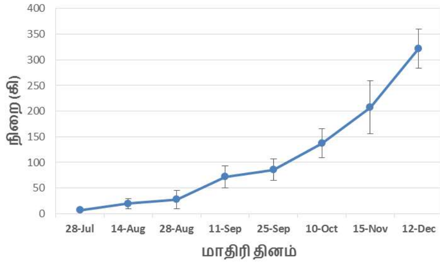
படம் 3: ரெக்கவ களப்பில் உள்ள வலைக் கூண்டுகளில் கடல் கொடுவா வளர்ப்பின் நீளம் (செமீ) மற்றும் நிறை (கிராம்) தரவுகளின் மாறுபாடு. கல்வி நோக்கங்களுக்காக ரெக்கவ களப்புப் பகுதியில் சதுப்புநில அடையாள பலகைகள் தயாரிக்கப்பட்டன.
