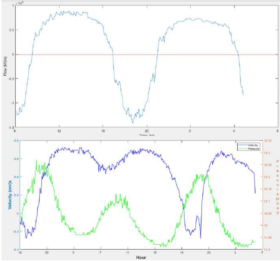
படம்20: மார்கழியில் தடாகத்தின் வாயில் அழுத்தத்துடன் நீர் ஓட்டம் வேகம்
