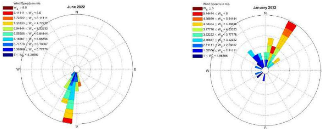
படம் 12 : தென்மேற்கு பருவமழை மற்றும் வடகிழக்கு பருவமழையின் போது காற்று அதிகரிப்பு வரைபடங்கள்.
