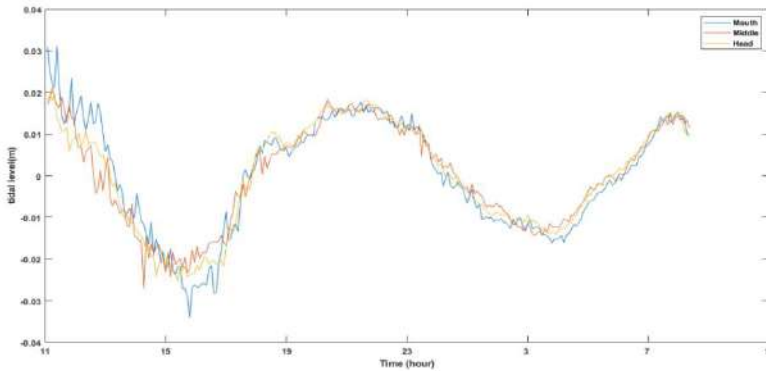
படம்14: ஜப்பசியில் களப்பின் கடல் மட்டத்தில் ஏற்ற இறக்கம்
