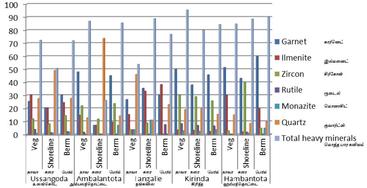
படம் 4: பருவமழைக்கு பின்னரான கனமான கனிம சதவீதம்
