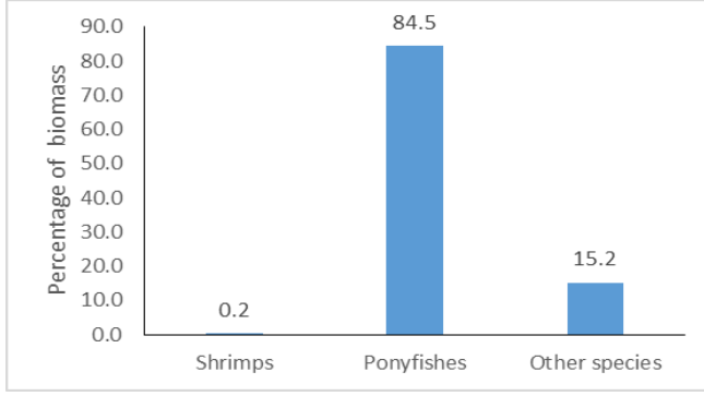
படம் 1. வரையறுக்கப்பட்ட இழுவைத் தளம் / கணக்கெடுப்புப் பகுதியில் உயிர்ப்பொருள் (%) விநியோகம் (N= மொத்த உயிர்ப்பொருள்)
