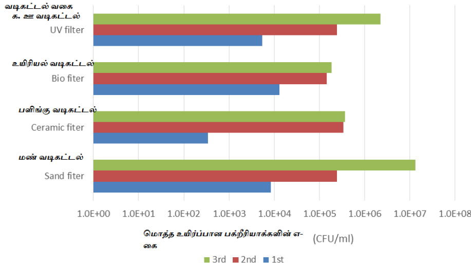
படம் 6: RAS அமைப்பின் மொத்த பக்றீரியா எண்ணிக்கை
