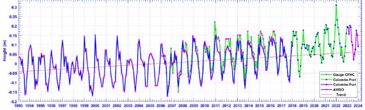
படம் 11: இலங்கையின் நீண்ட கால கடல் மட்ட அவதானிப்புகளை படம் காட்டுகிறது.
