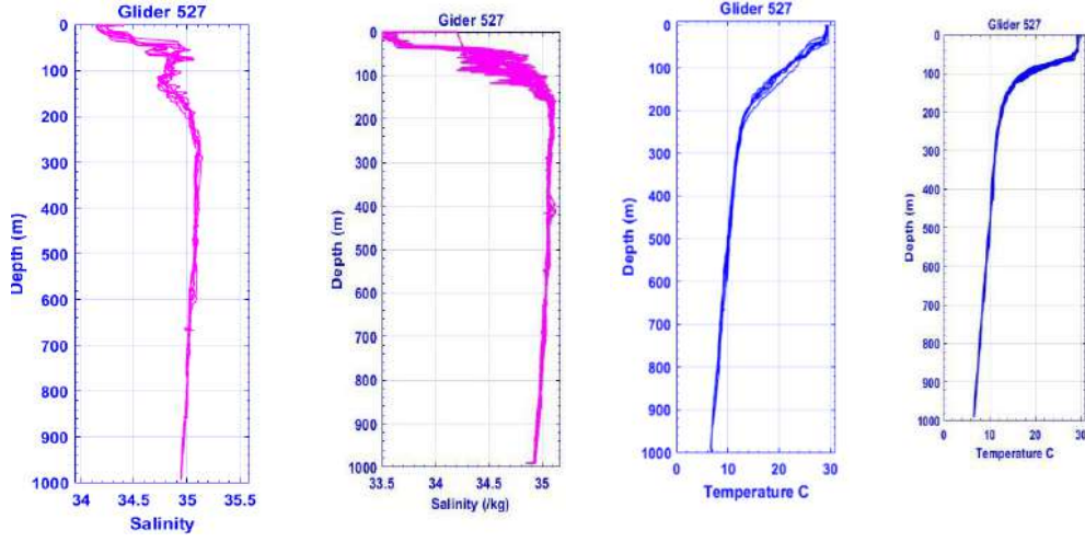
படம் 15 : தென்மேற்கு பருவமழையின் போது உப்புத்தன்மை மற்றும் வெப்பநிலை மாறுபாடு.
