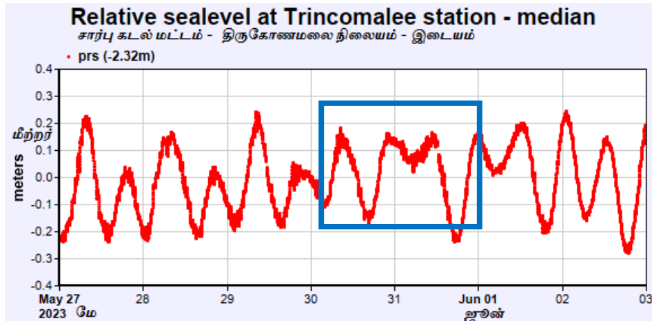
படம்11: வைகாசி மாதம் ஆய்வின் போது திருகோணமலையில் கடல் மட்டத்தில் ஏற்ற இறக்கம்
