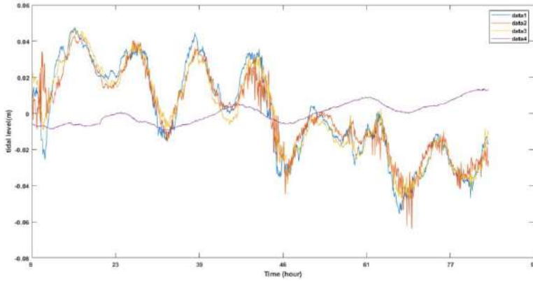
படம்12: மாவணி மாதத்தில் களப்பில் அலை ஏற்ற இறக்கம்
