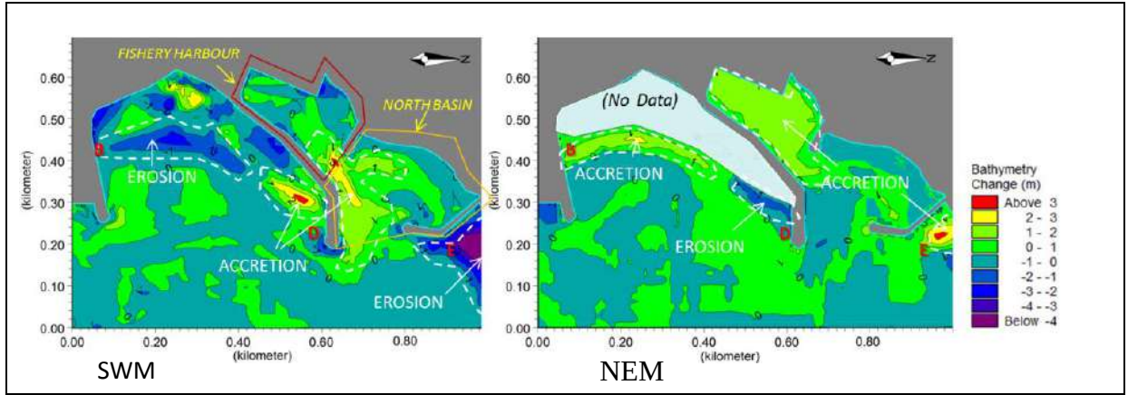
படம் 5: தென்மேற்கு பருவமழை (இடது) மற்றும் வடகீழ் பருவமழை (வலது) போது அளவிடப்பட்ட வண்டல் அரிப்பு விநியோகம் (லக்நாத், 2011)
