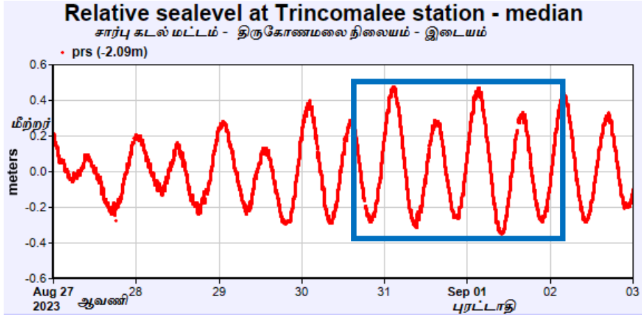
படம்13: ஆவணி மாதம் ஆய்வின் போது திருகோணமலையில் அலை மாற்றம்
