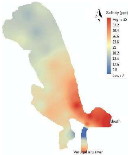
படம் 24: வைகாசி மாதத்தில் ம உப்புத்தன்மை மாறுபாடு
