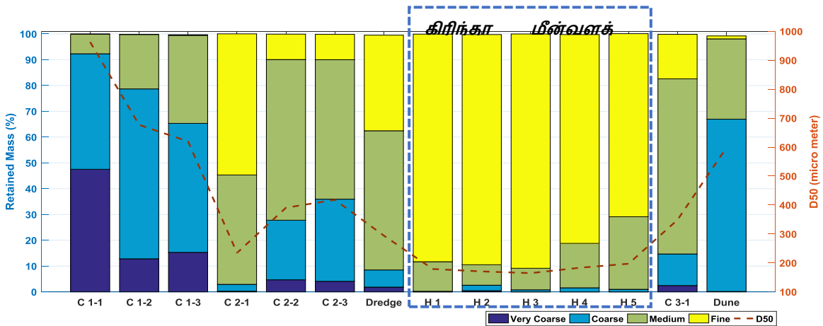
படம் 6: கரையோரத்தில் வண்டல் மாதிரிகள் தக்கவைக்கப்பட்ட நிறை (%) மற்றும் நடுத்தர துகள் அளவு (D50). மிகவும் கரடுமுரடான (>1 மி.மீ), கரடுமுரடான (1 மி.மீ - 0.5 மி. மீ), நடுத்தர (0.5 மி.மீ - 0.25 மி. மீ) மற்றும் மெல்லிய மணல் (<0.25 மி. மீ)
