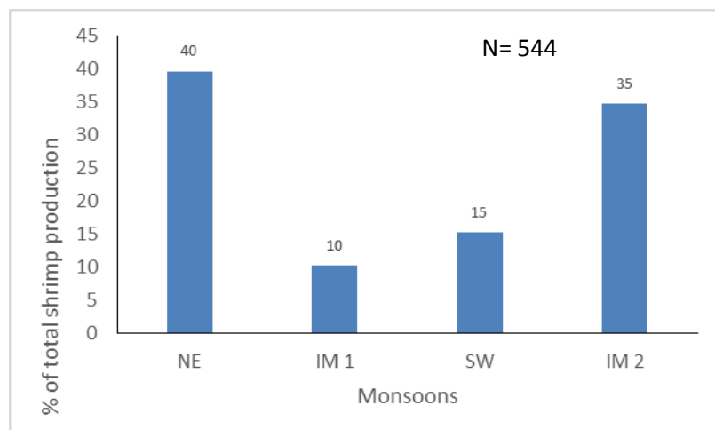
படம் 4. மொத்த இறால் உற்பத்தியின் பருவகால ஏற்ற இறக்கம் கல்பிட்டி டிராமல் வலை மீன்பிடி வளம்
