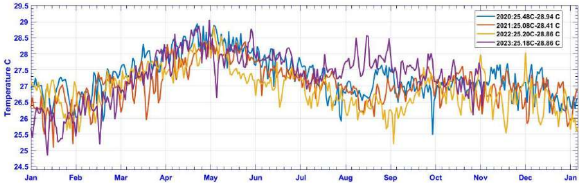
படம் 14 : இலங்கையின் தெற்கு கடற்கரையில் வெப்பநிலை மாறுபாடு.
