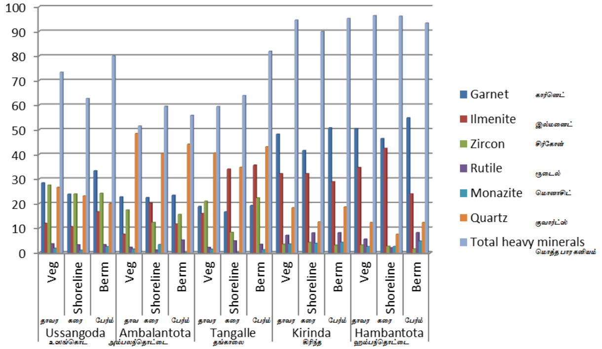
படம் 03 : பருவமழைக்கு முந்தைய கனமான கனிம சதவீதம்
