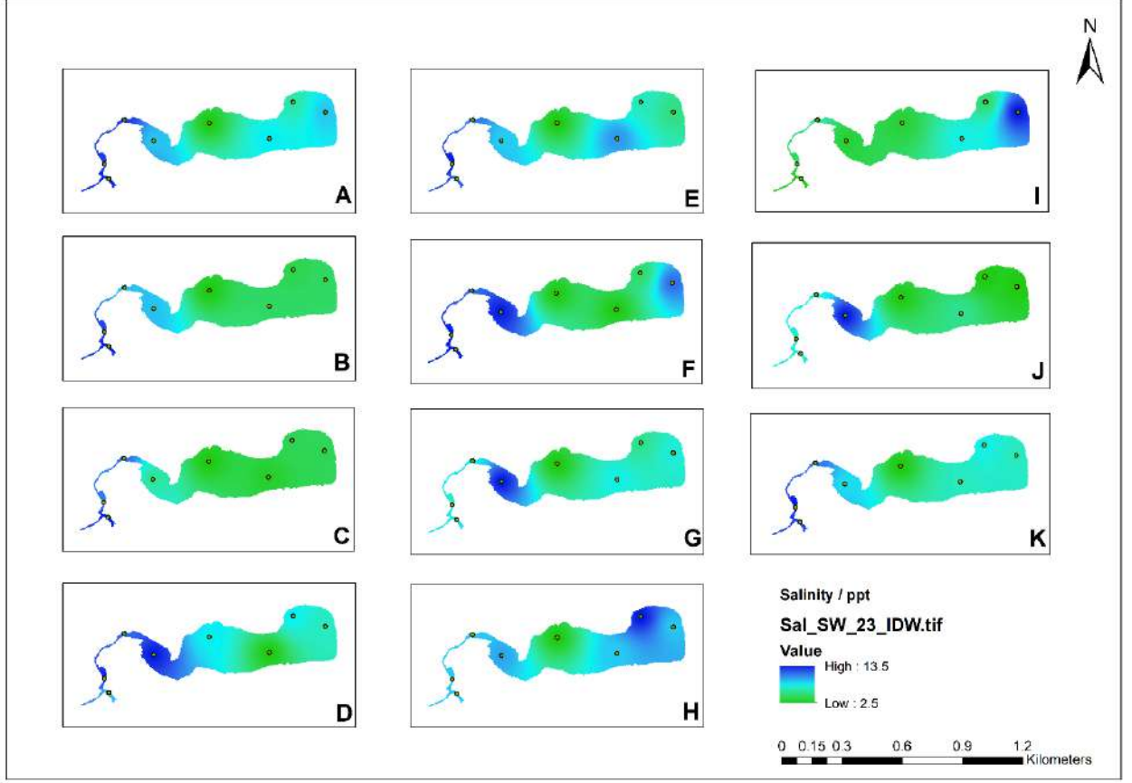
படம் 1: ரெக்கவ களப்பின் உப்புத்தன்மை விநியோக வரைபடங்கள் (A: வ. கீ பருவக்காற்று, 2021; B: 1IM, 2021; C: த்.மே பருவக்காற்று, 2021; D: 2IM, 2021; E: வ. கீ பருவக்காற்று, 2022; F: 1IM; 2022IM; ஜி: தெ.மே பருவமழை, 2022; 2IM, 2022; I: வ.கீ பருவக்காற்று, 2023; K: தெ. மே பருவக்காற்று, 2023)
