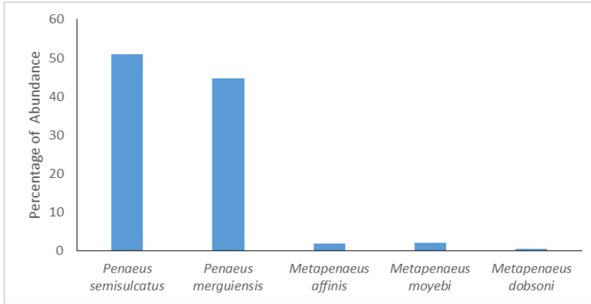
படம் 2. கல்பிட்டி இழுவைத் தளத்தில் பதிவுசெய்யப்பட்ட இறால் இனங்களில் மிகுதியான (%) மாறுபாடு
