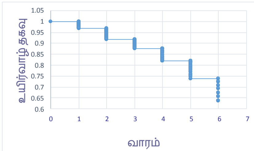
படம் 2: கலப்பின நபர்களின் உயிர்வாழும் நிகழ்தகவின் மாறுபாடு.
