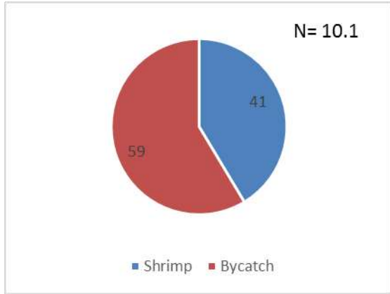
படம் 3. கல்பிட்டி டிராமல் வலை மீன்பிடி வளத்தின் வருடாந்த சராசரி CPUE இன் கலவை சதவீதம்
