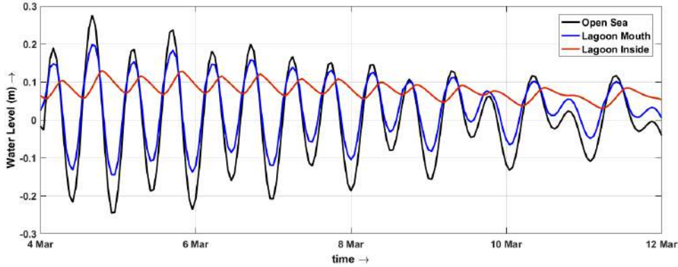
படம்34: லங்காபட்டுன களப்பு வாய் மற்றும் திறந்த கடல் ஆகியவற்றில் உள்ள நீர் நிலை மாறுபாடுகள்
