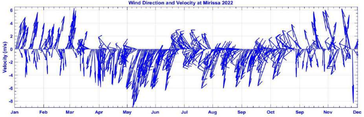
படம் 13:காற்றின் திசை மற்றும் அலைவீச்சின் நேரத் தொடர் கண்காணிப்பு.
